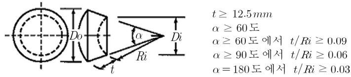
그림 1.5.4 (a) 원볼테두리 구상 부채형 관망창
