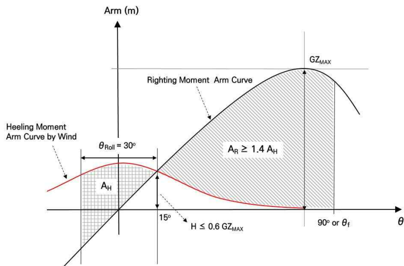
그림 8 횡풍에 의한 횡동요 상태에서의 비손상 복원정 및 경사우력정 곡선
