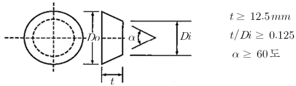
그림 1.5.2 원볼형 절두체 관망창
