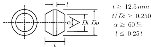
그림 1.5.3 이중 경사판식 관망창
