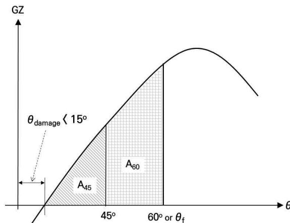
그림 9 잠수선의 손상 복원정 곡선
