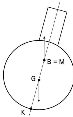
그림 3 수중에서의 GM(=GB)
