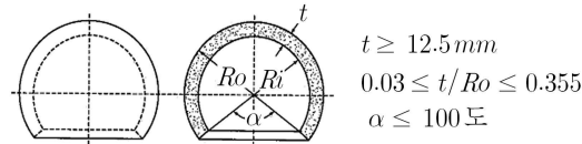
그림 1.5.4 (b) 초반구형 관망창
