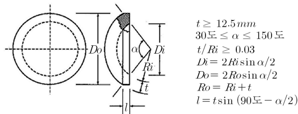
그림 1.5.5 (a) 사각 테두리 구상 부채형 관망창
